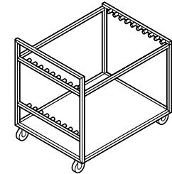
546/90 Transportwagen zur Aufnahme von fünf Klappptischen 540/25 (Tischtiefe 90 cm)
